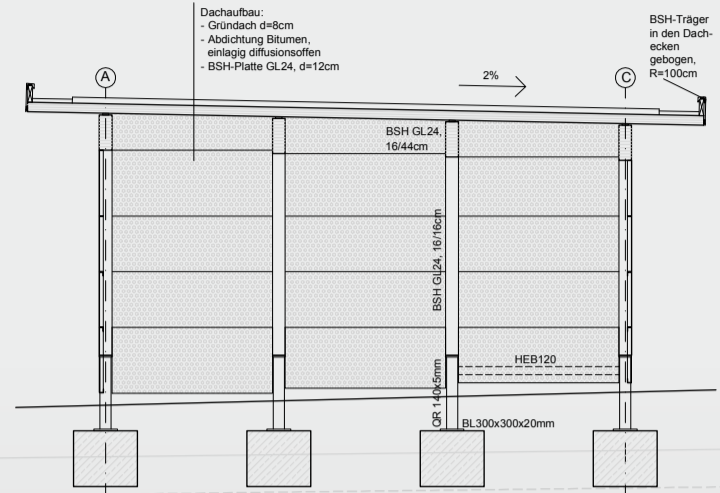
A Schnitt A
