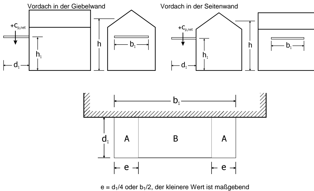
Bild 1 — Abmessungen und Einteilung der Flächen für Vordächer
