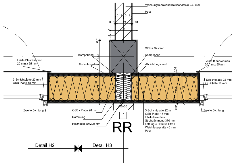
Detail - Anschluss Außenwand
