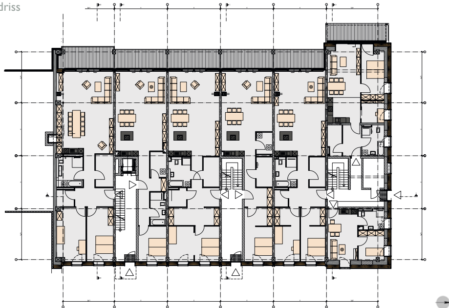
Grundriss
