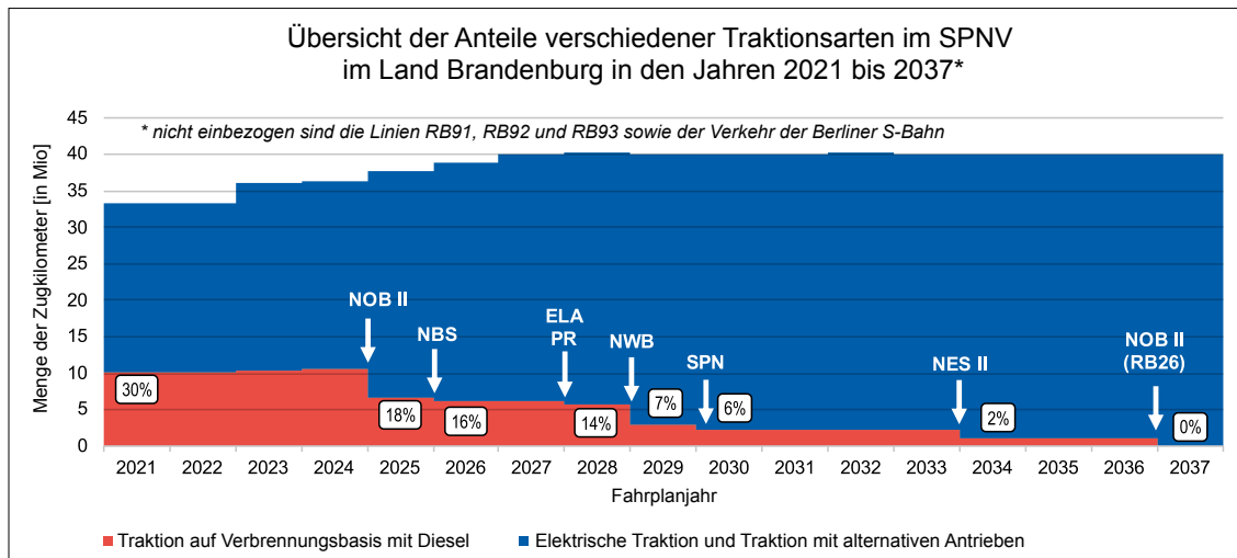
Abbildung 8: Übersicht der Anteile verschiedener Traktionsarten im SPNV im Land Brandenburg in den Jahren 2021-2037 (Quelle: VBB GmbH)
