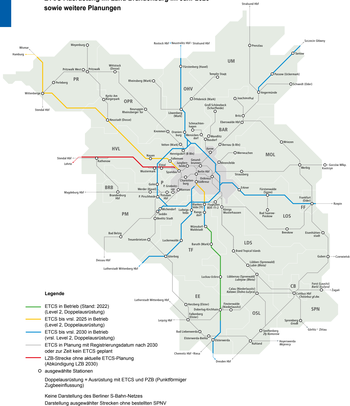
Karte 4: Aktueller und geplanter Infrastruktur-Ausrüstungsstand mit dem Zugsicherungssystem ETCS im Land Brandenburg mit Stand Februar 2023 (Quelle: VBB GmbH)
