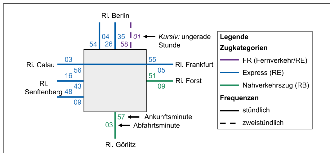
Abbildung 6: Beispiel eines integralen Taktknotens (Cottbus Hbf/Chósebusz Główny, Stand: 3. Gutachterentwurf Zielfahrplan Deutschlandtakt) (Quelle: SMA und Partner AG)
